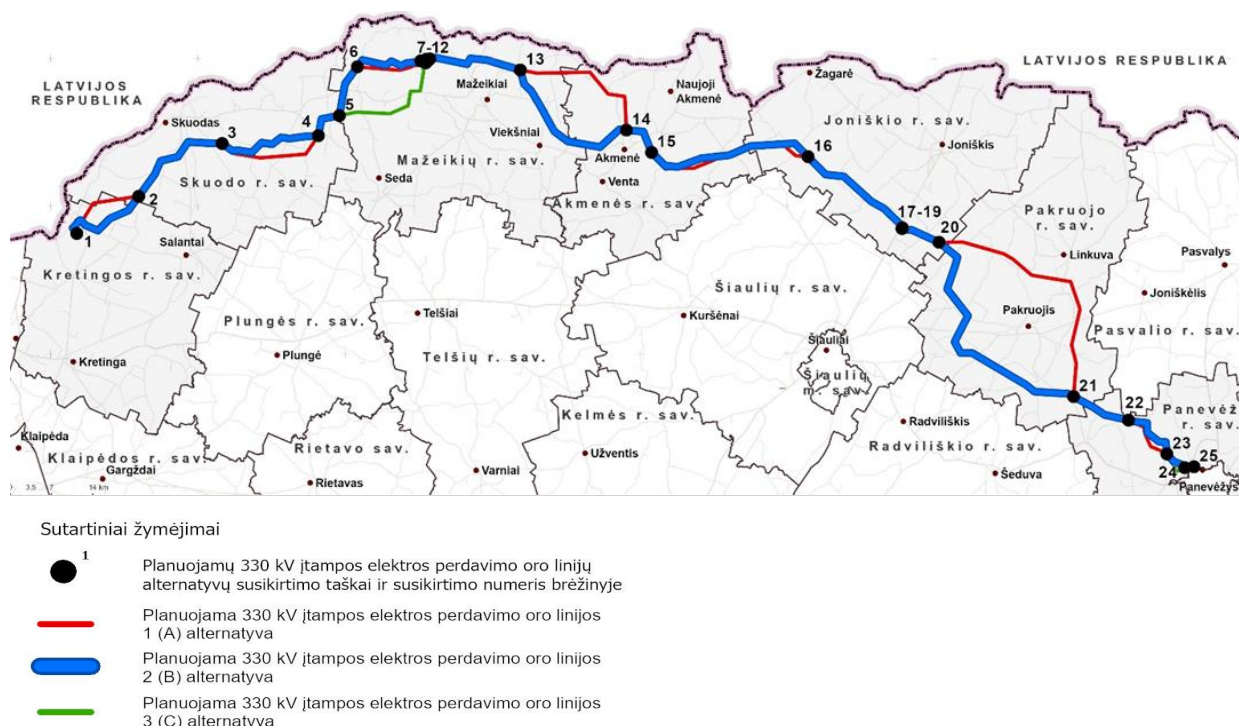
5 pav. Preliminarios 330 kV elektros perdavimo oro linijos trasos alternatyvos (B) schema
