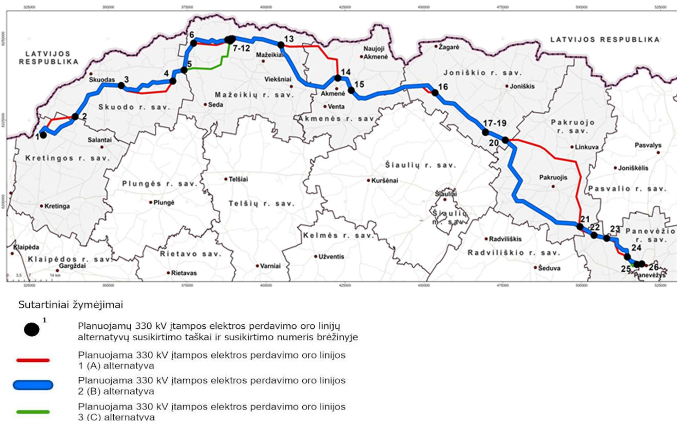
5 pav. Preliminarios 330 kV elektros perdavimo oro linijos trasos alternatyvos (B) schema
