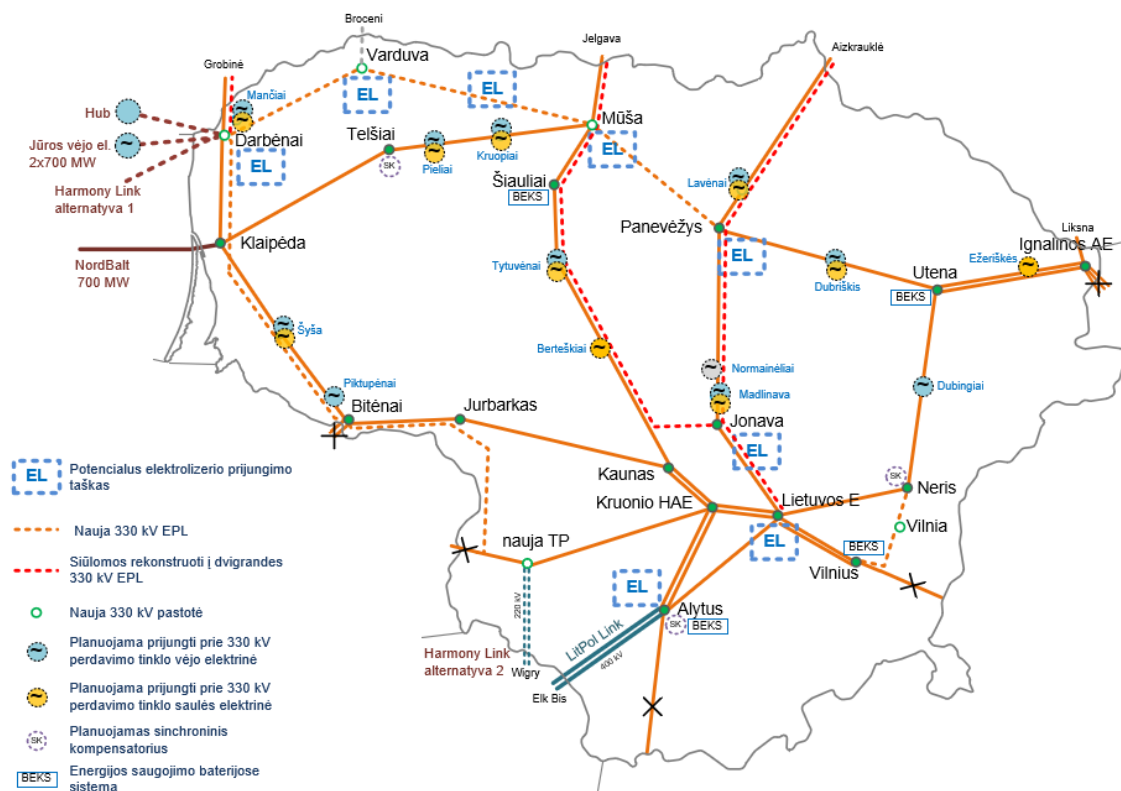
1 pav. 400-330 kV perdavimo tinklas 2033 m. (Šaltinis: AB „Litgrid“ „Lietuvos elektros energetikos sistemos 400-110 kV tinklų plėtros planas 2024-2033 m.“)
