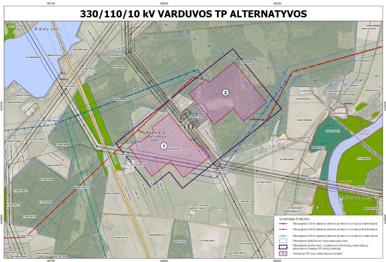
7 pav. Varduvos TP alternatyvų principinė schema
