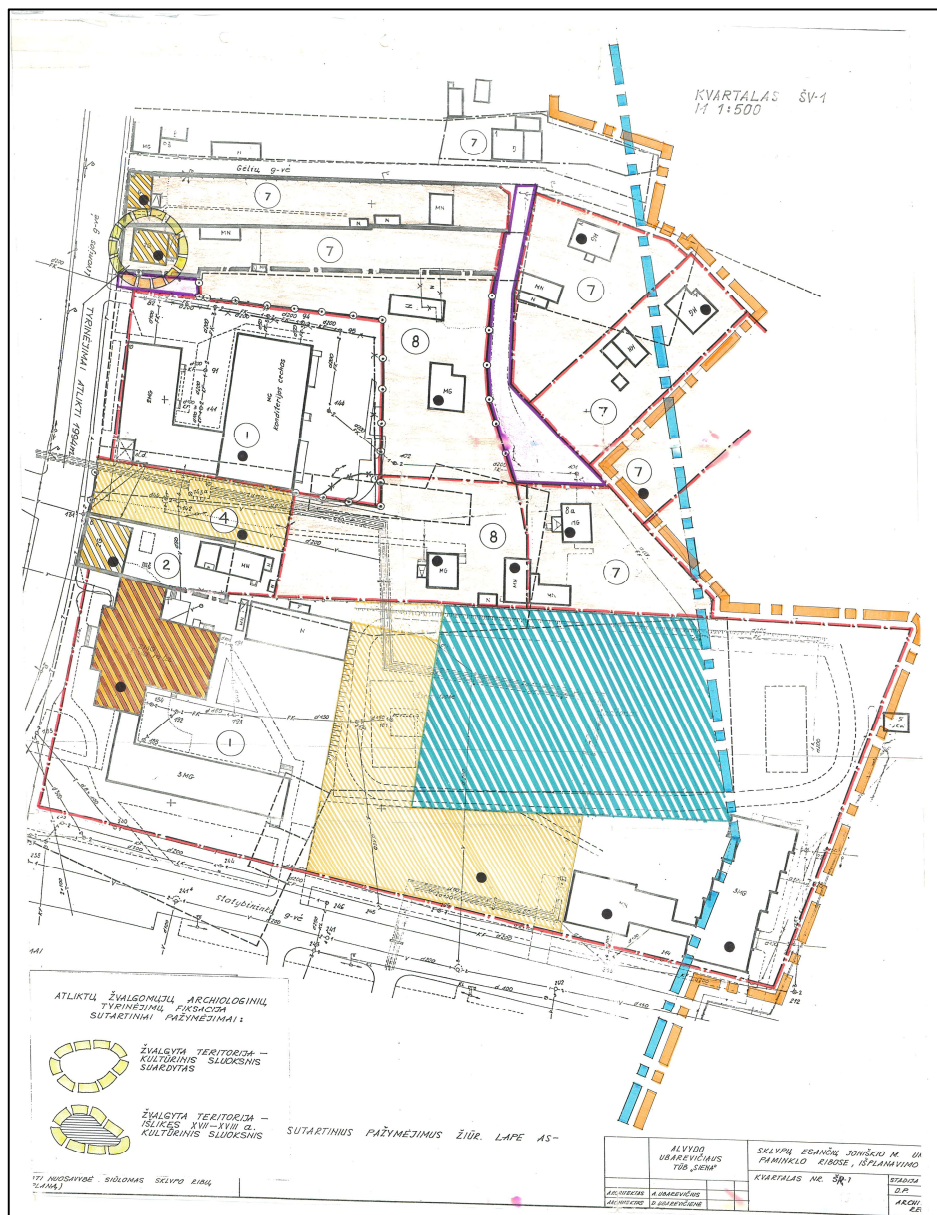
8 pav. Ištrauka iš teritorijų planavimo dokumento: Vietinės reikšmės Urbanistikos paminklo UV-15 Joniškio mieste sklypų suplanavimo projektas. „Kvartalas ŠV-1 M 1:500“ detalizacija (šaltinis: www.tpdri.lt ).
