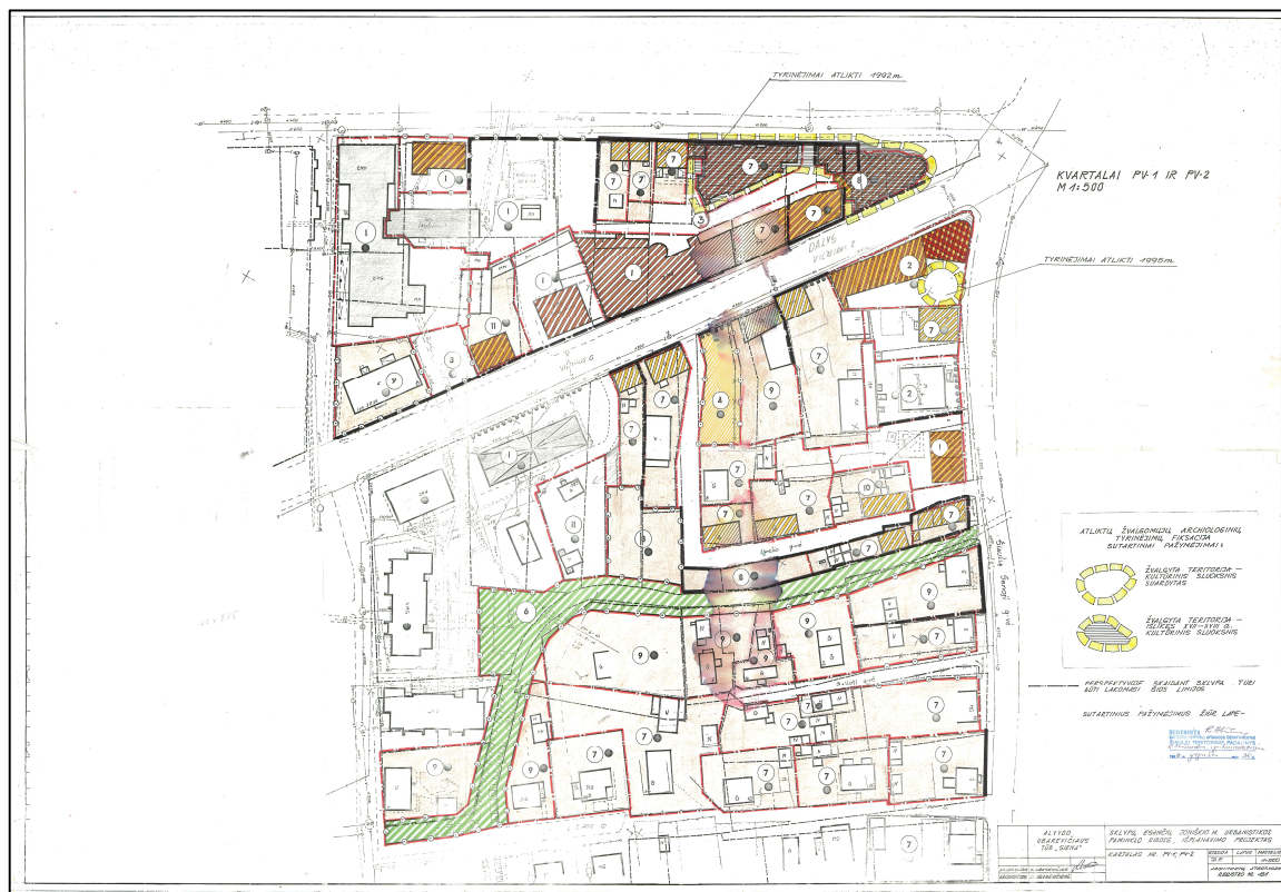
4 pav. Ištrauka iš teritorijų planavimo dokumento: Vietinės reikšmės Urbanistikos paminklo UV-15 Joniškio mieste sklypų suplanavimo projektas. „Kvartalai Nr. PV-1 ir PV-2 M 1:500“ detalizacija (šaltinis: www.tpdri.lt).
